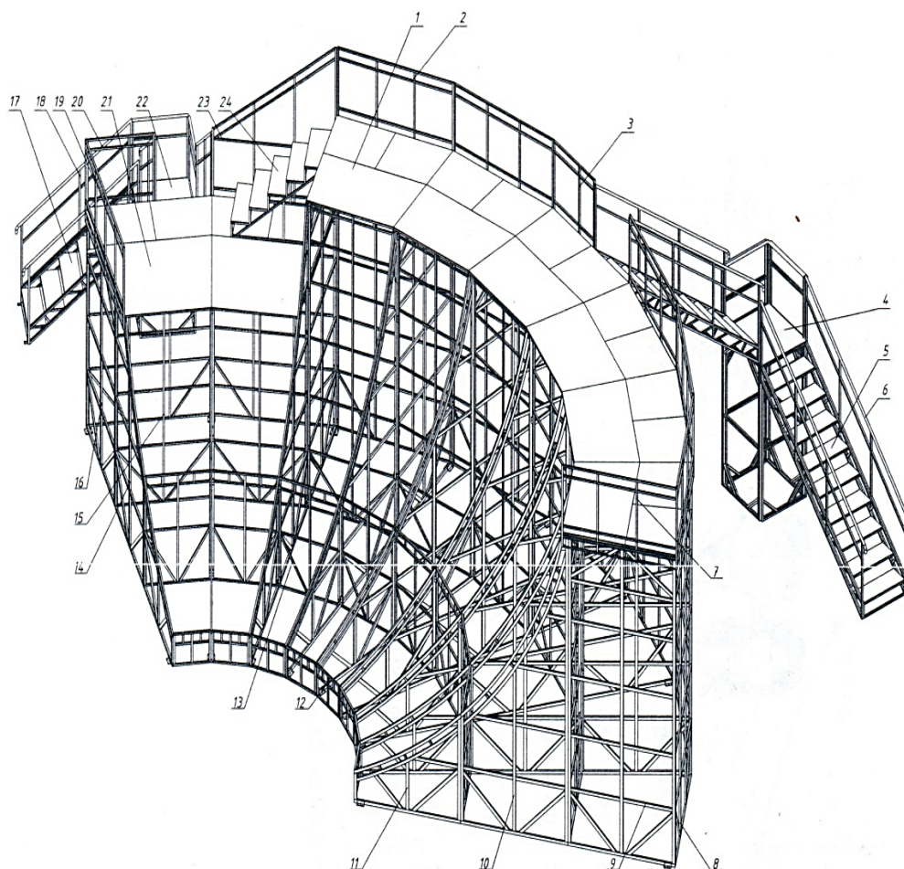
Рис. 3.2 Рабочий станок
